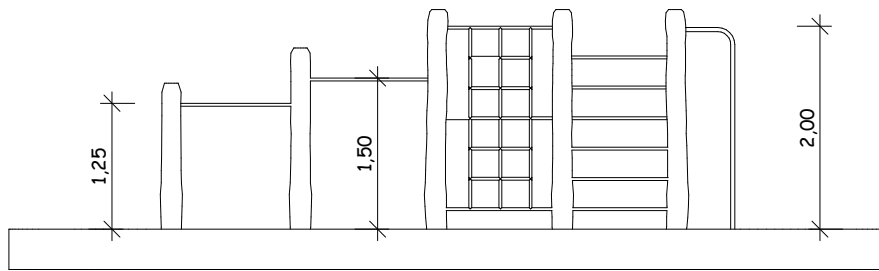
Ansicht
